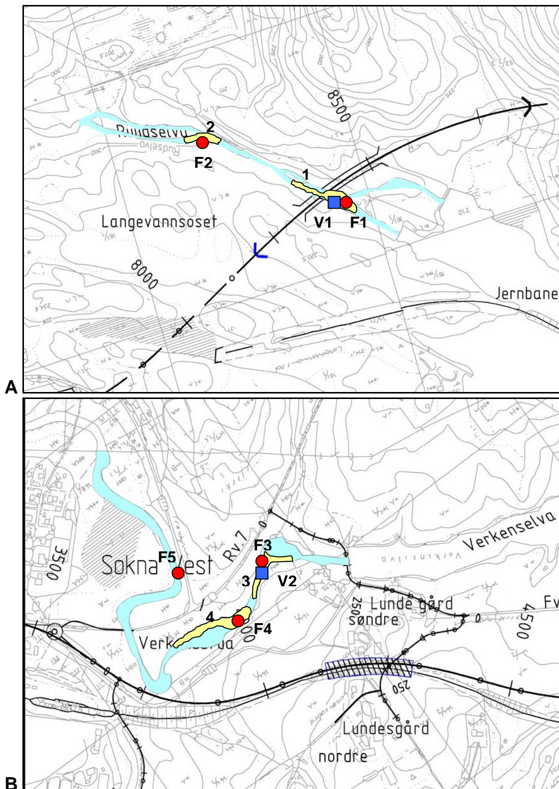
Figur 5. Illustrasjonsplan for veitraséen med kryssningspunkt med Rudselva (A) og nærføring til Verkenselva (B). Undersøkte elvestrekninger er markert med lys blå farge. Lokalisering av vannprøvestasjoner (V1-V2, blå firkant), elfiskestasjoner (F1-F5, rød sirkel) og elvemuslingstasjoner med fritelling (1-4, gult areal) er vist. Kartgrunnlag gjengitt med tillatelse fra Statens vegvesen.
