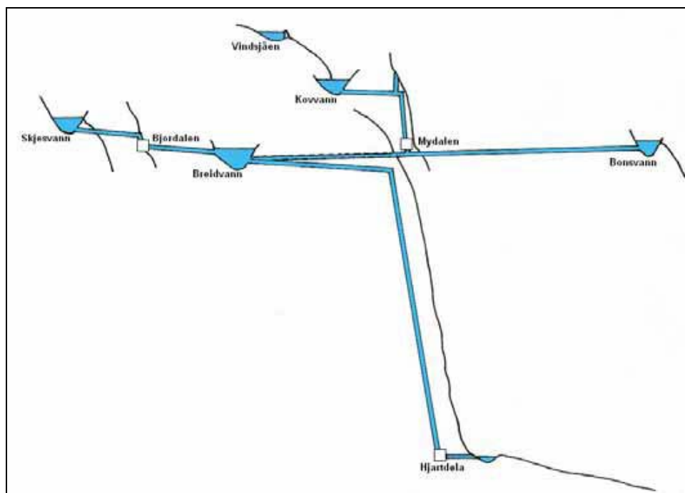
Figur 2.2. Eksisterende magasin og kraftverk i Hjørdals- og Tuddalsvassdraget
