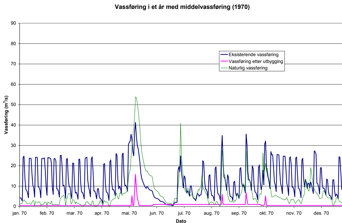
Figur 3.2. Vannføringsvariasjon nedenfor inntaket til Sauland 1 i året nærmest middelvannføring. Figuren er basert på verdier med døgnoopløsning, slik at de sterke endringene i løpet av uken ved eksisterende vannføring er synlige.
