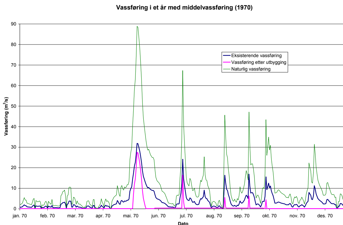
Figur 3.4. Vannføringsvariasjon nedenfor inntaket til Sauland 2 i året nærmest middelvannføring: naturlig vannføring, eksisterende vannføring (med Hjartdøla kraftverk) og etter utbygging av Sauland kraftverk
