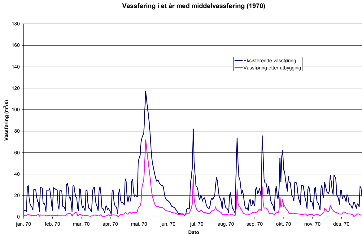
Figur 3.5. Vannføringsvariasjon ved Omnesfossen umiddelbart oppstrøms utløpet fra Sauland kraftverk i året nærmest middelvannføring, før og etter utbygging.
