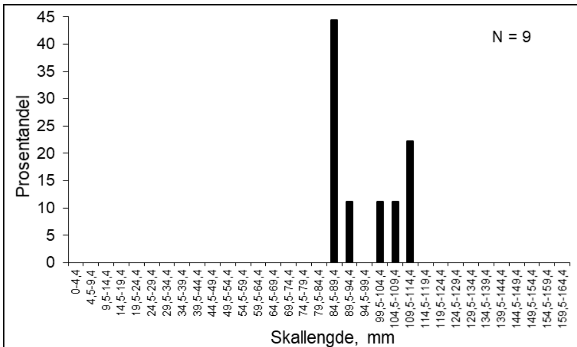
Figur 5.5. Lengdefordeling av levende elvemusling fra Lilleelv i 2019.
