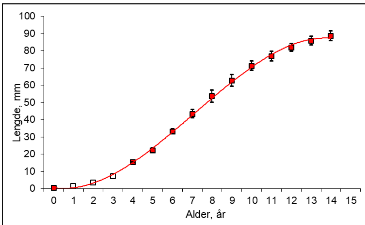
Figur 5.6. Vekstkurve basert på lengde av gjennomsnittlig årringsdiameter hos aldersbestemte elvemusling i Lilleelv fram til 14 års alder (N=2). Figuren viser gjennomsnittlig, maksimum og minimum lengde for hver alder, i tillegg til estimert vekstkurve. Lengder ved 1-3 års alder er hentet fra data fra Oгна i Rogaland (Larsen mfl. 2012).
