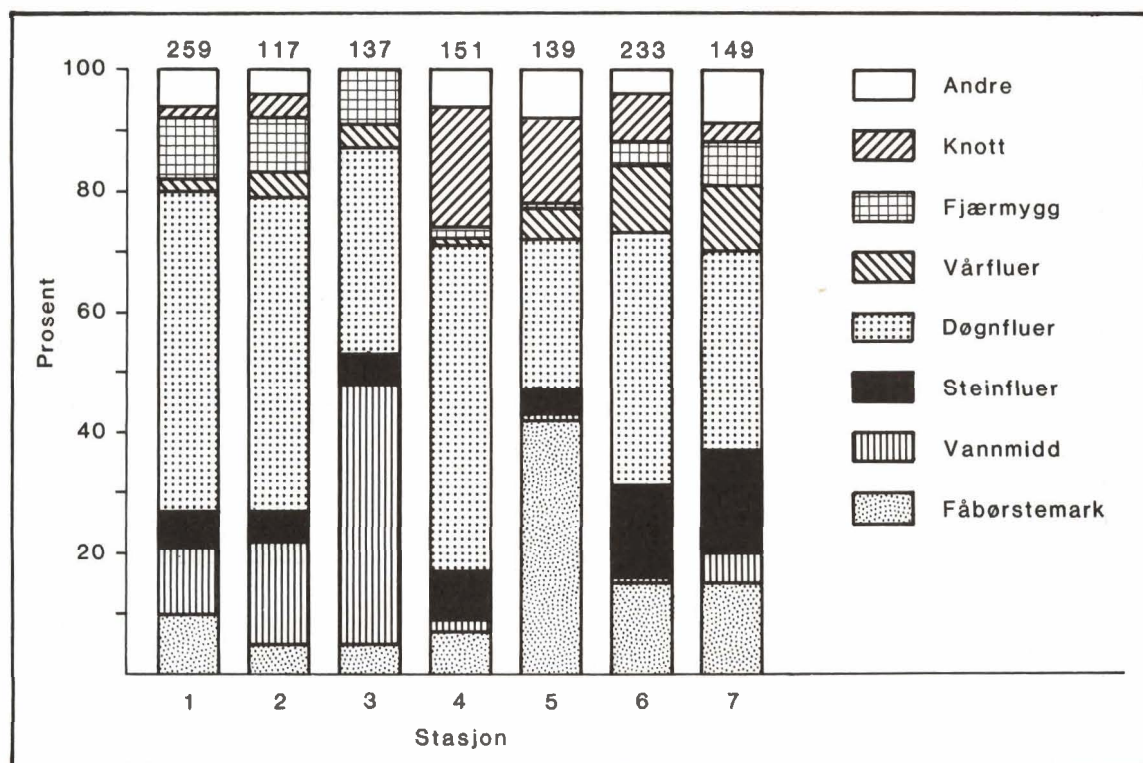
Figur 2. Prosentvis sammensetning av bunnfaunaen på de forskjellige stasjonene i Homla. Sammensetningen er basert på prøver tatt i oktober 1985 og juni 1986. Gjennomsnittlig antall bunndyr pr. 1 min. sparkeprøve er angitt på toppen av søylene.
