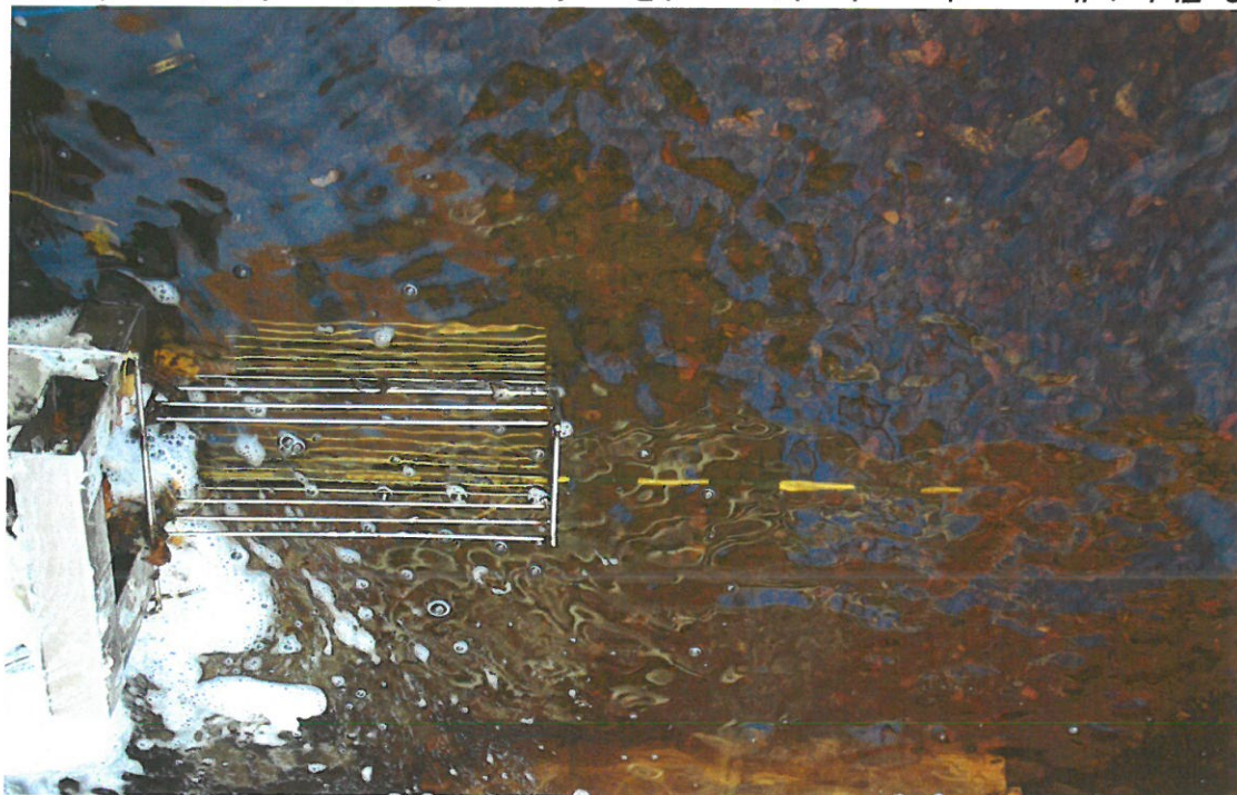
Figur 2. Fisketellerens plassering i trappa i Berrefossen. Lengden på fisken måles mot målestaven montert på kalven som står i forlengelsen av selve tellerkanalisen.
