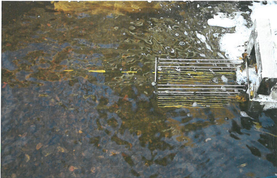
Figur 2. Fisketelleren i trappa i Berrefossen. Lengden på fisken måles mot målestaven montert på kalven som står i forlengelse av selve tellemekanismen.
