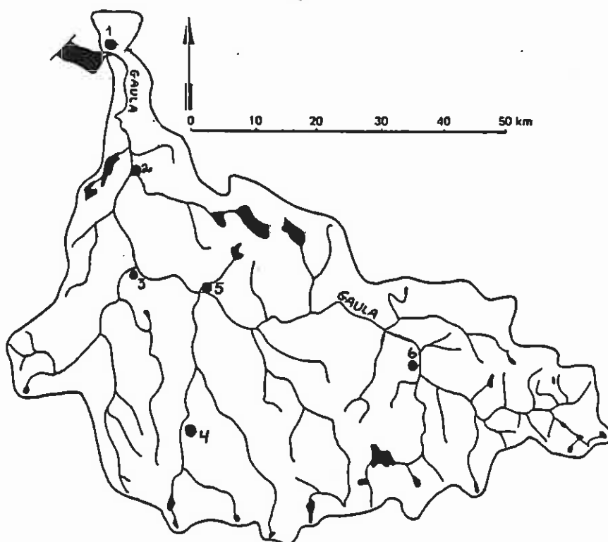
Figur 2. Nedbørstasjoner i Gaulas nedbørfelt.
